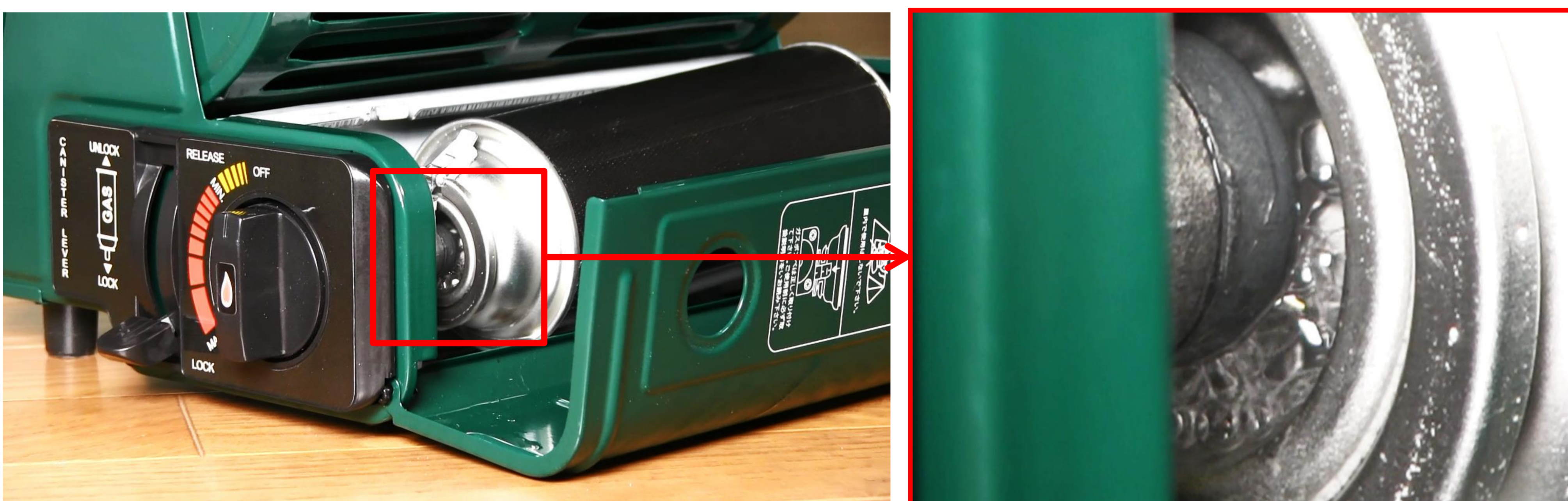
正しく装着されずに、カセットボンベ式ガスストーブとボンベの隙間からガスが漏れている様子(イメージ)
